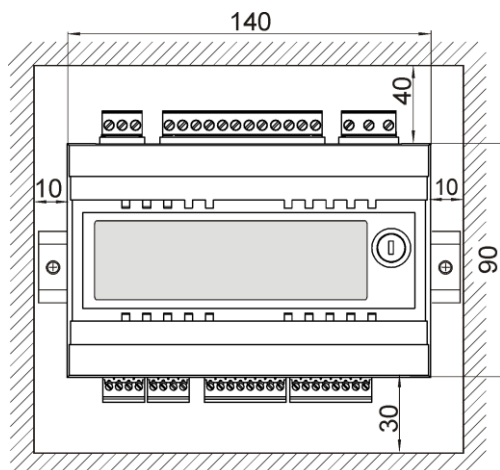
Условия монтажа модуля.
